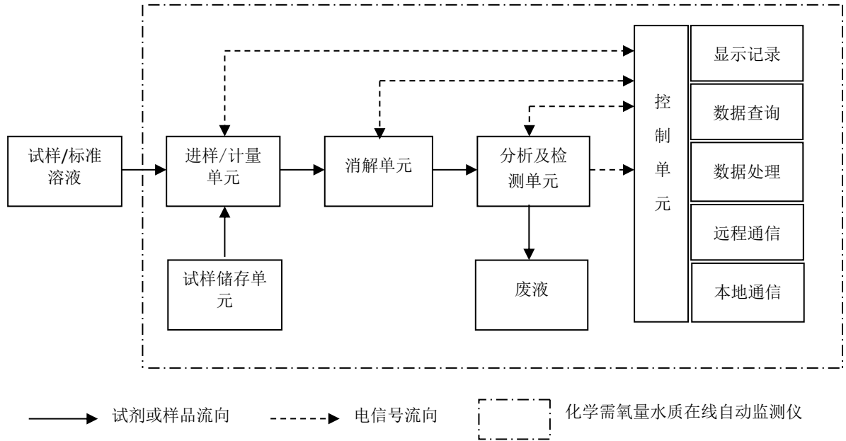
图 1 化学需氧量（COD Cr ）水质在线自动监测仪的基本组成单元
